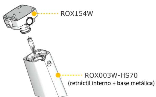
ROX154W
