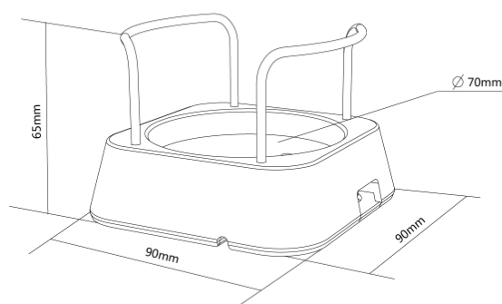
Soporte de exhibición para ópticas FOX821
