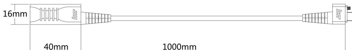
Cable de conmutación para corriente alta (Cable obligatorio para cada sensor de carga seleccionado si se ha seleccionado un adaptador de 12 V para el controlador)
