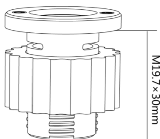
Φ20 Conjunto de fijación (30mm) FOX180-30
