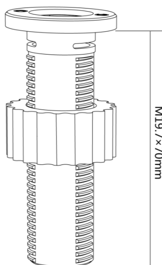
Φ20 Conjunto de fijación (70mm) FOX180-70
