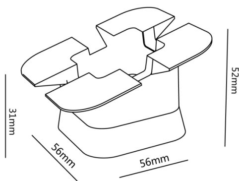
Soporte horizontal 15° Tablet FOX712
