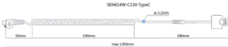
Cable rizado blanco de carga conector Type C SEN614W-C130-TypeC
