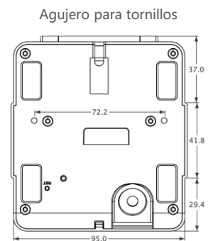
iBox090T vista inferior
