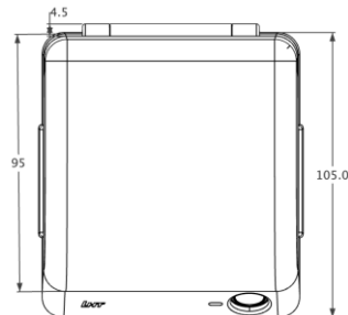
iBox090T vista superior
